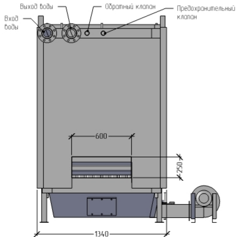
Котел водогрейный КВр-0,35 ДВО:
