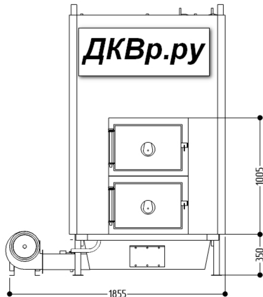
Котел водогрейный КВр-0,63 ДВО:
