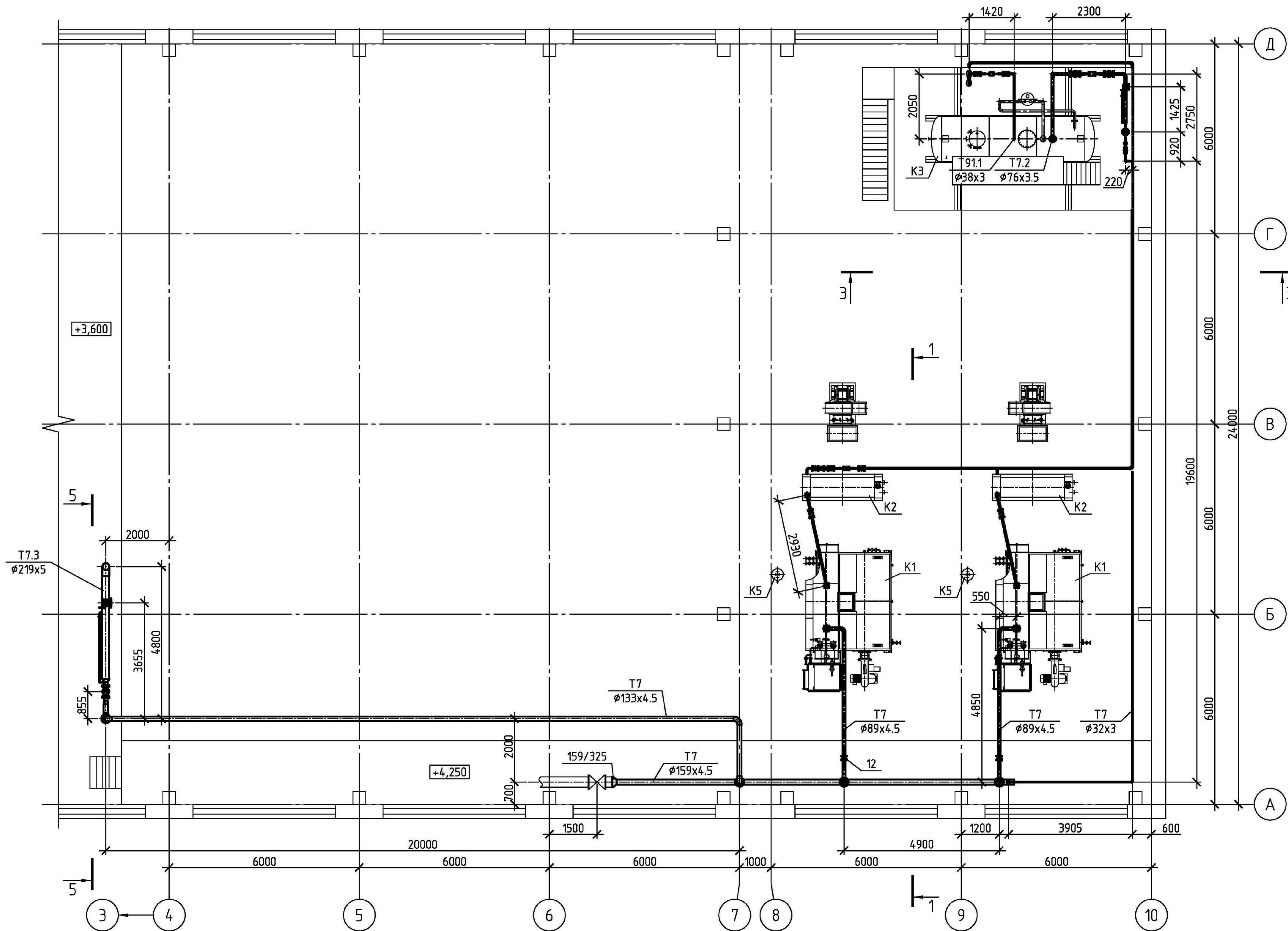
План на отм +4.250
