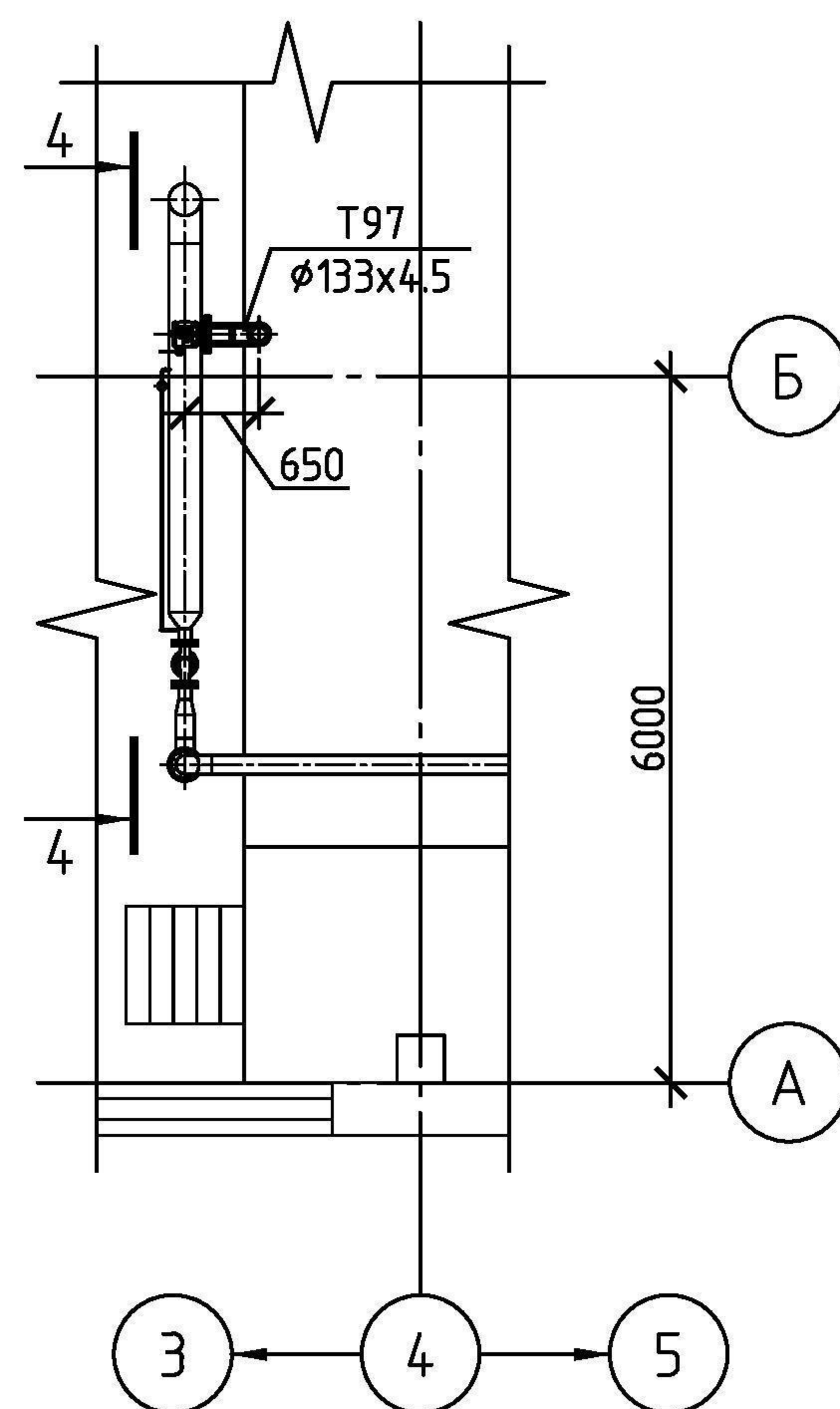
План на отм +4.250
