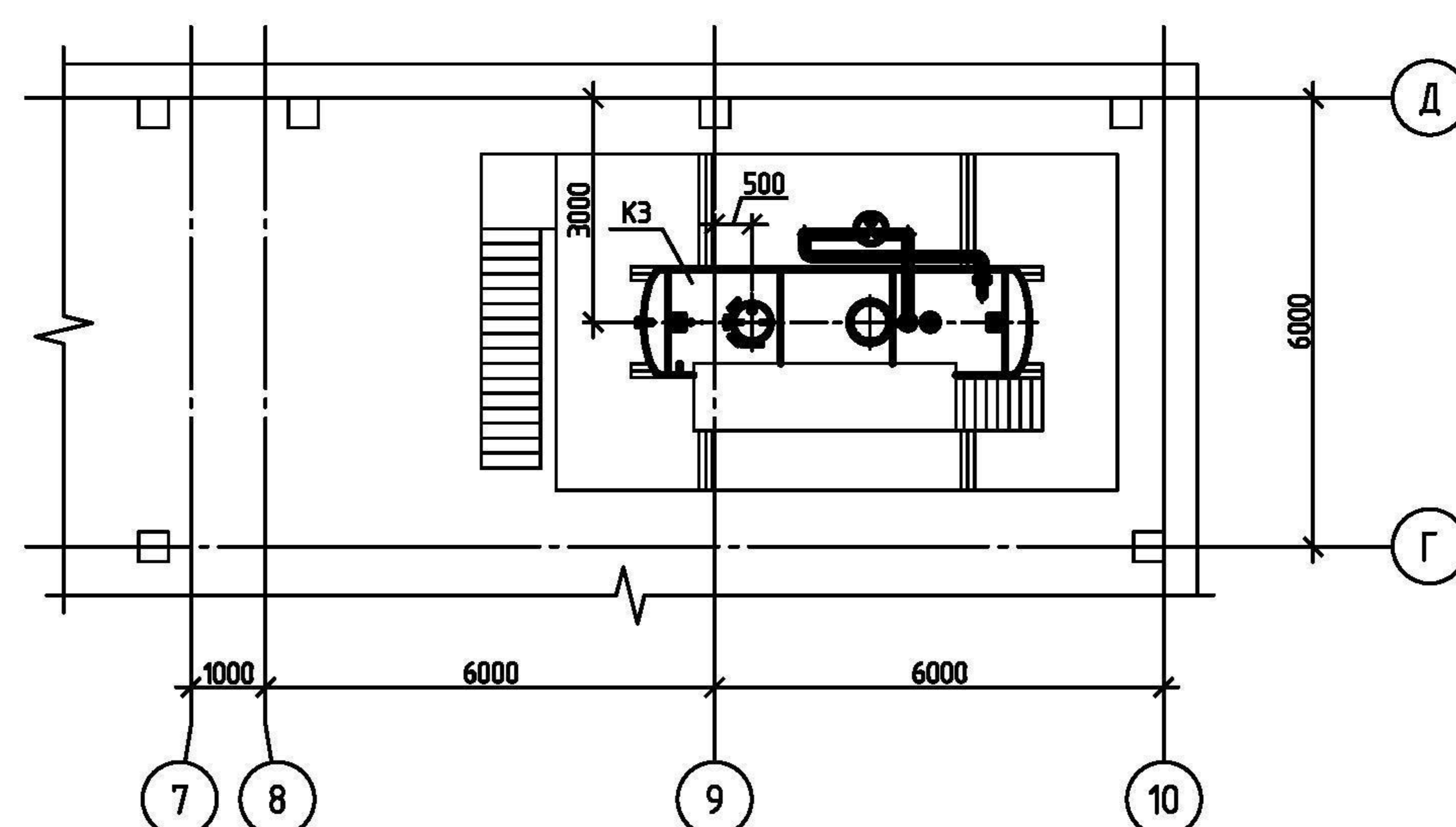
План на отм +4.250
