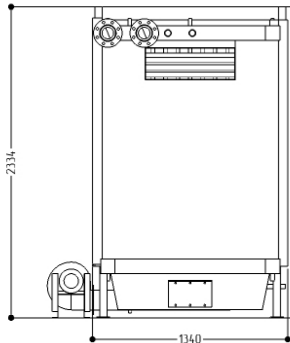
Котел водогрейный КВа-0,8:
