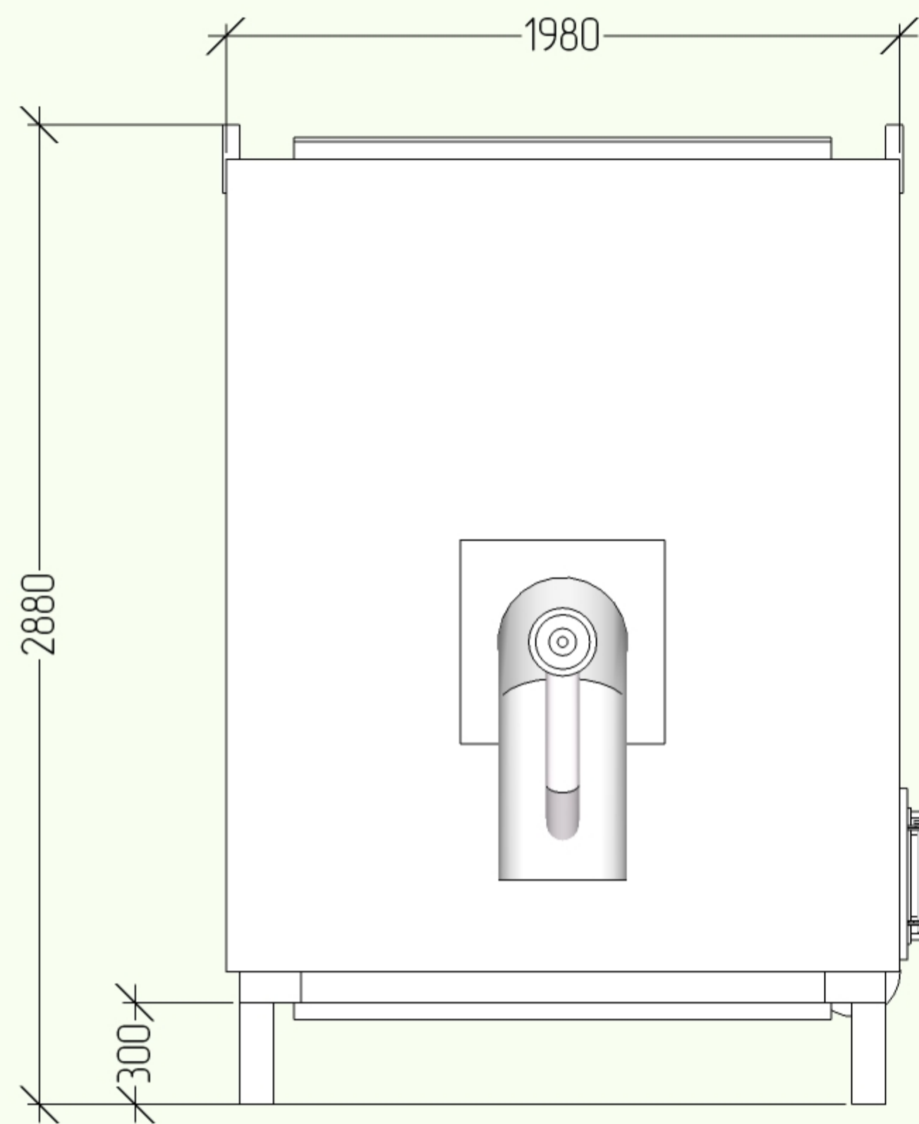
Котел водогрейный КВа-2,5:
