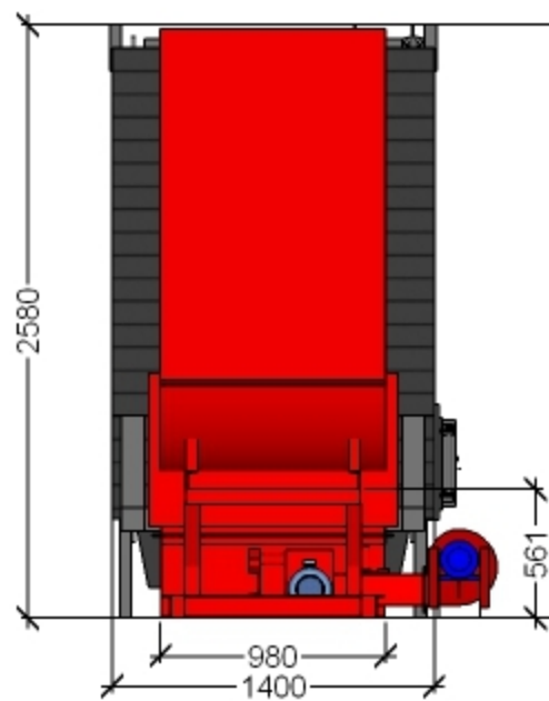
Котел водогрейный КВм-1,5:
