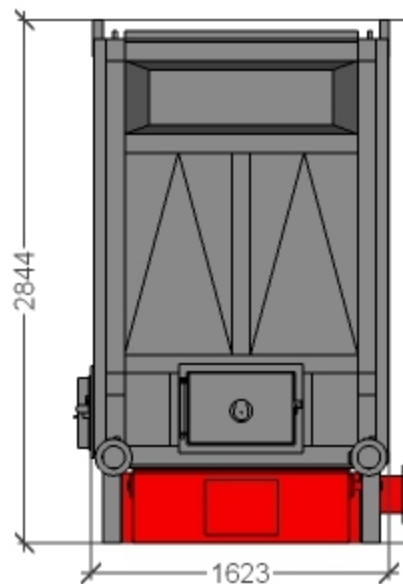
Котел водогрейный КВи-3,0:
